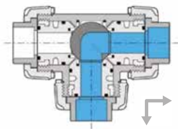
L-boring 90° open positie 2
