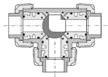
L-boring 180° gesloten positie 2
